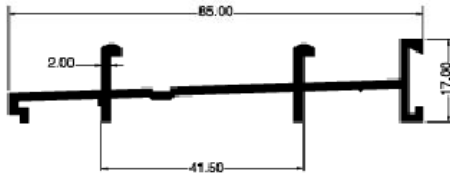
8025-1 UMBRAL BRONCE 5.8 MTS
