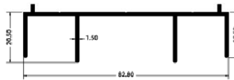
8025-2 CARGADOR BRONCE 5.8 MTS
