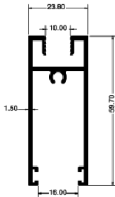
8025-4 HOJA INFERIOR BRONCE 5.8 MTS
